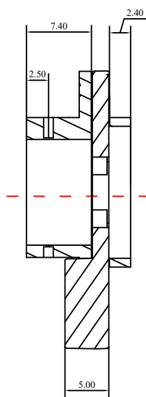
剖面A-A
